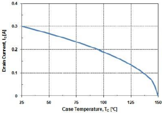
Fig. 9 I_D - T_C
